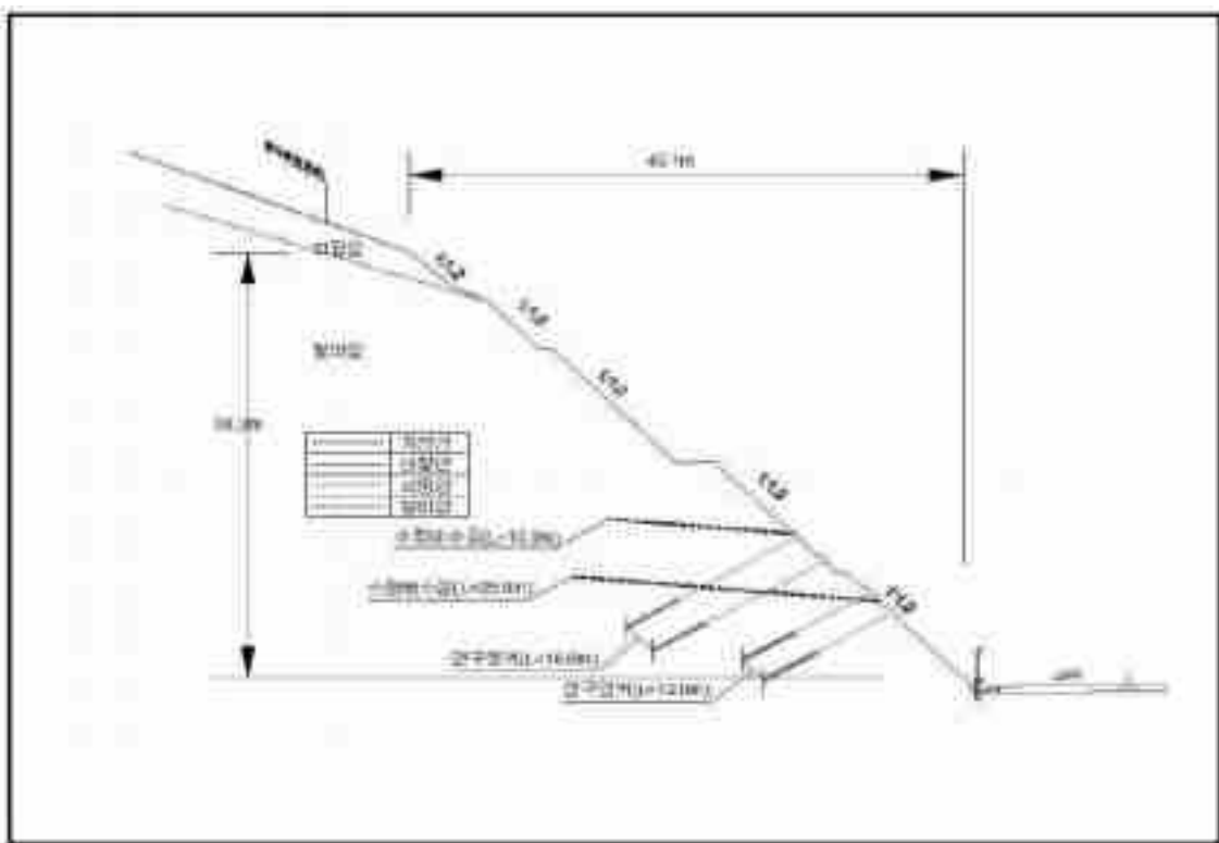
【대표단면 Stn.3+140(상주)】
