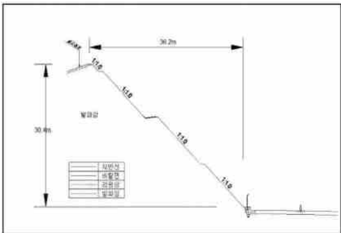
【대표단면 Sta.6+220(상주)】
