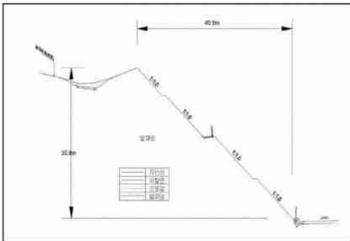
【대표단면 Sta.5+300(상주)】
