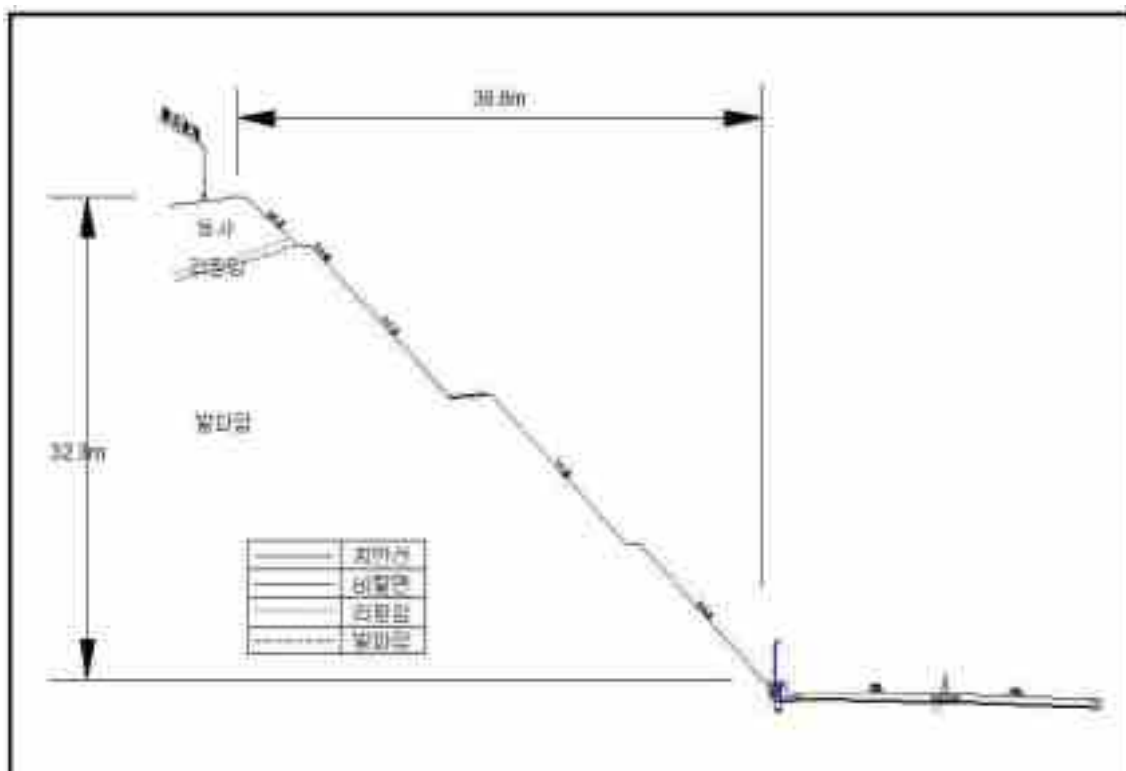
【대표단면 Sta.6+360(상주)】
