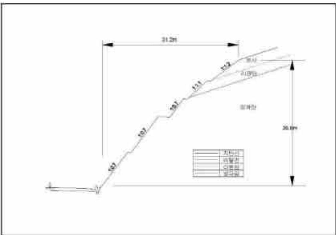
【대표단면 Sta.0+700(영원)】
