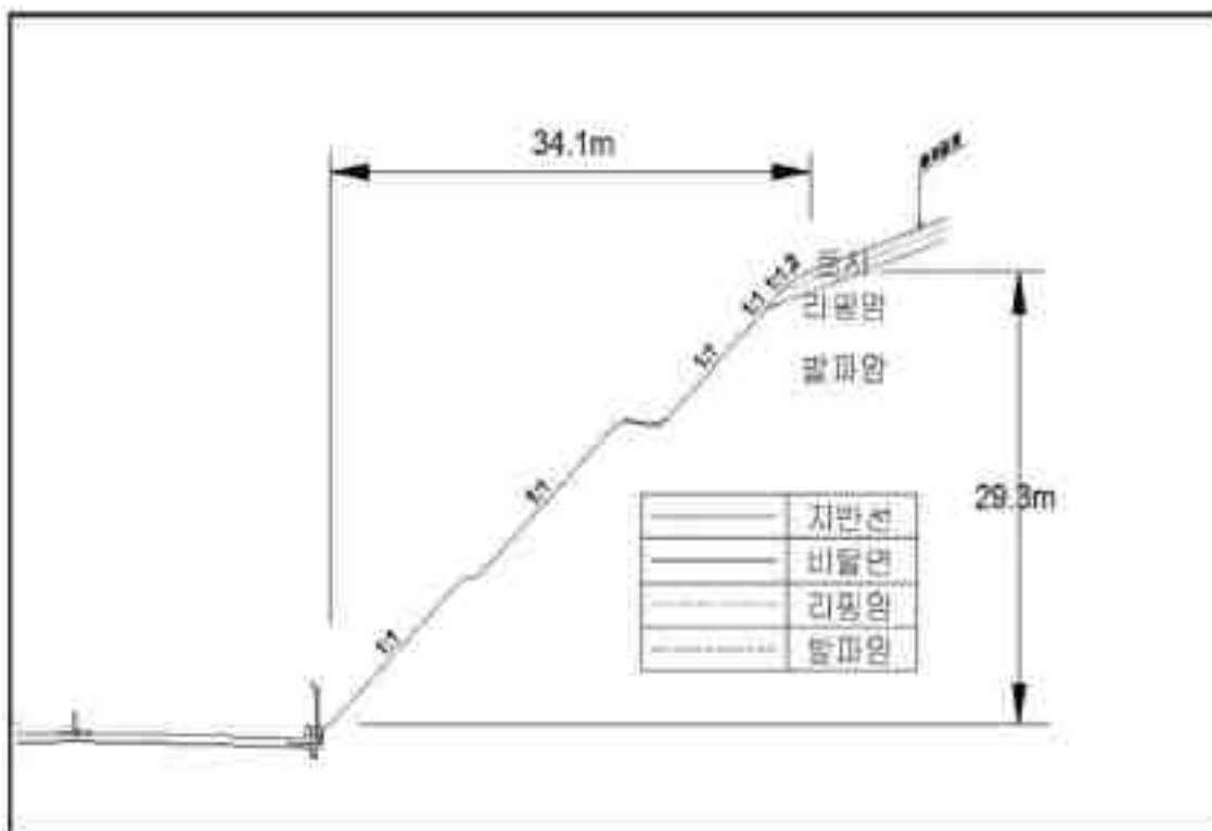
【대표단면 Sta.9+500(영원)】
