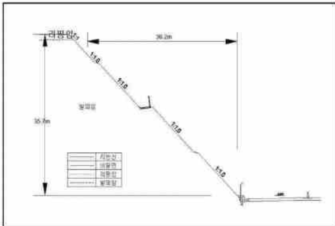
【대표단면 Sta.9+680(상부)】
