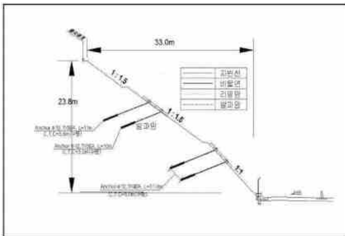
【대표단면 Sta.5+780(상주)】
