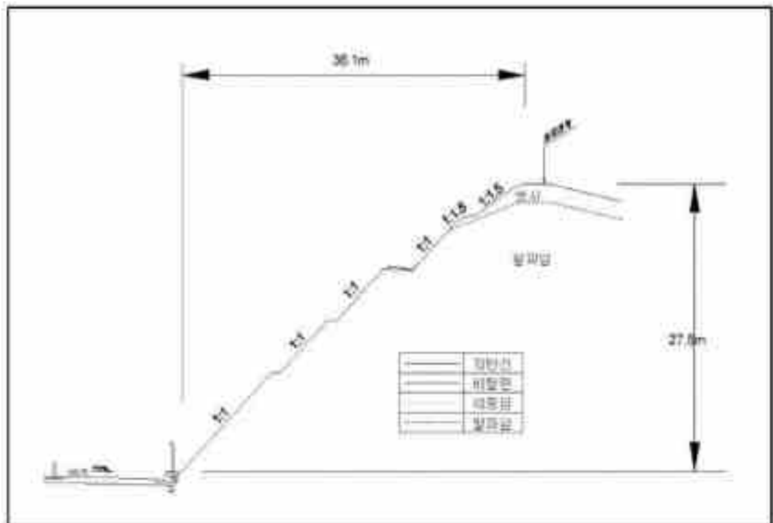
【대표단면 Sta.4+800(영천)】
