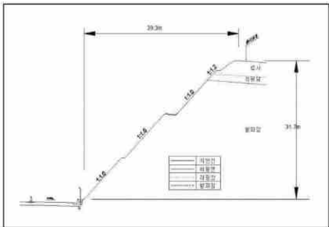
【대표단면 Sta.3+820(영천)】
