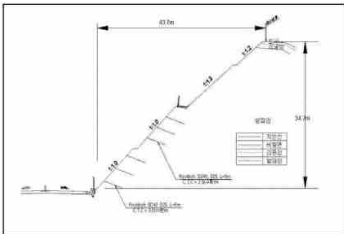
【대표단면 Sta.4+800(영원)】
